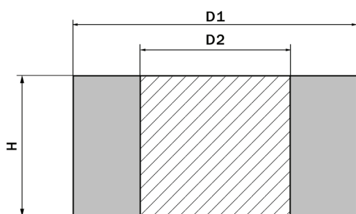
Rysunek przekroju tulei gumowej
